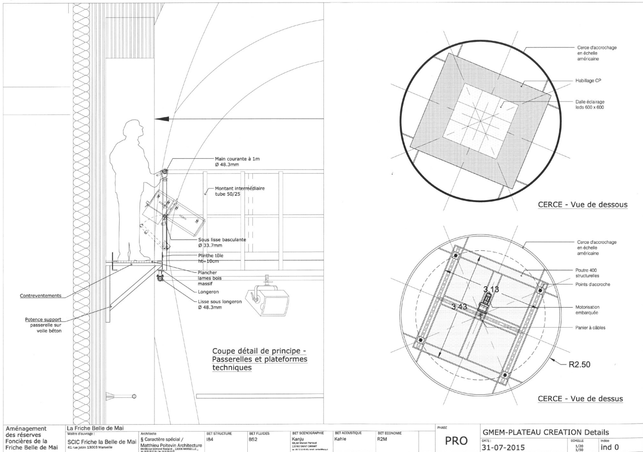
Détail des passerelles
